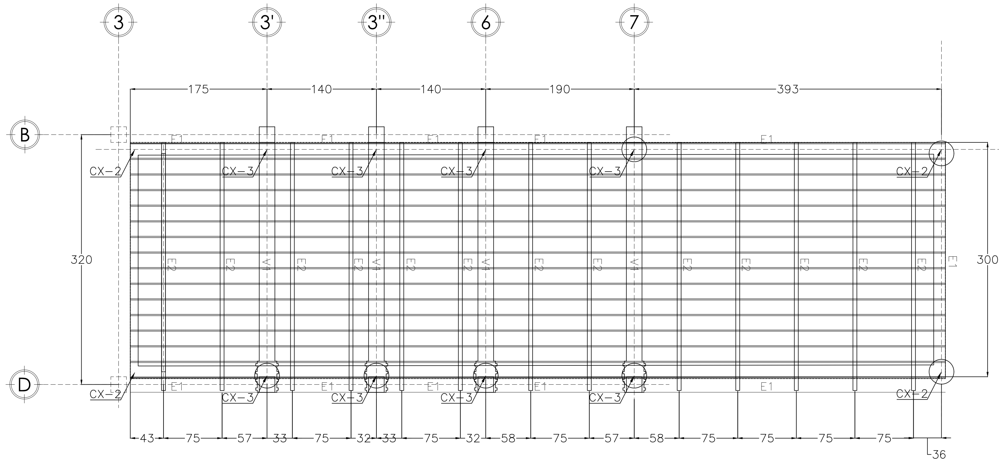
PLANTA DE CUBIERTA METÁLICA 1 Acot: mm
