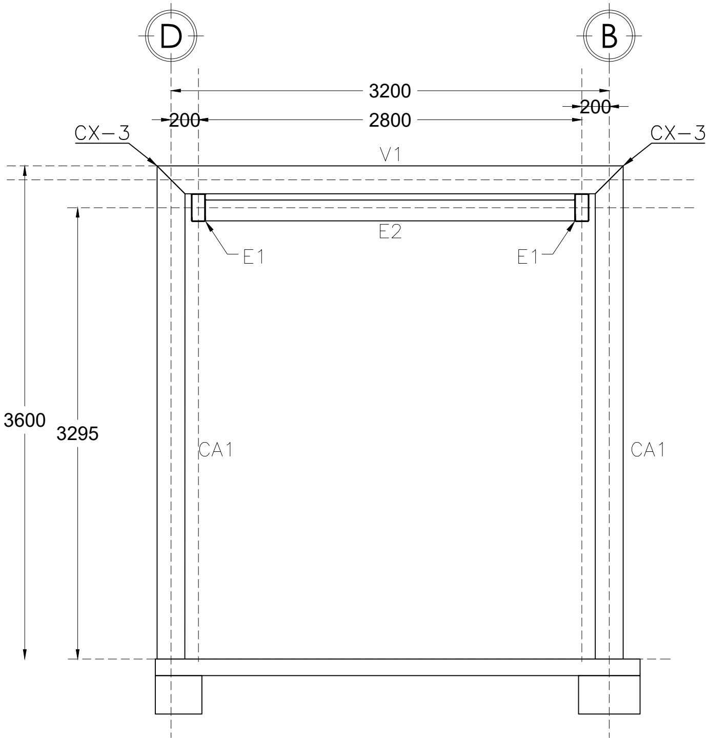
MARCO TRANSVERSAL CUBIERTA 1 Acot: mm
