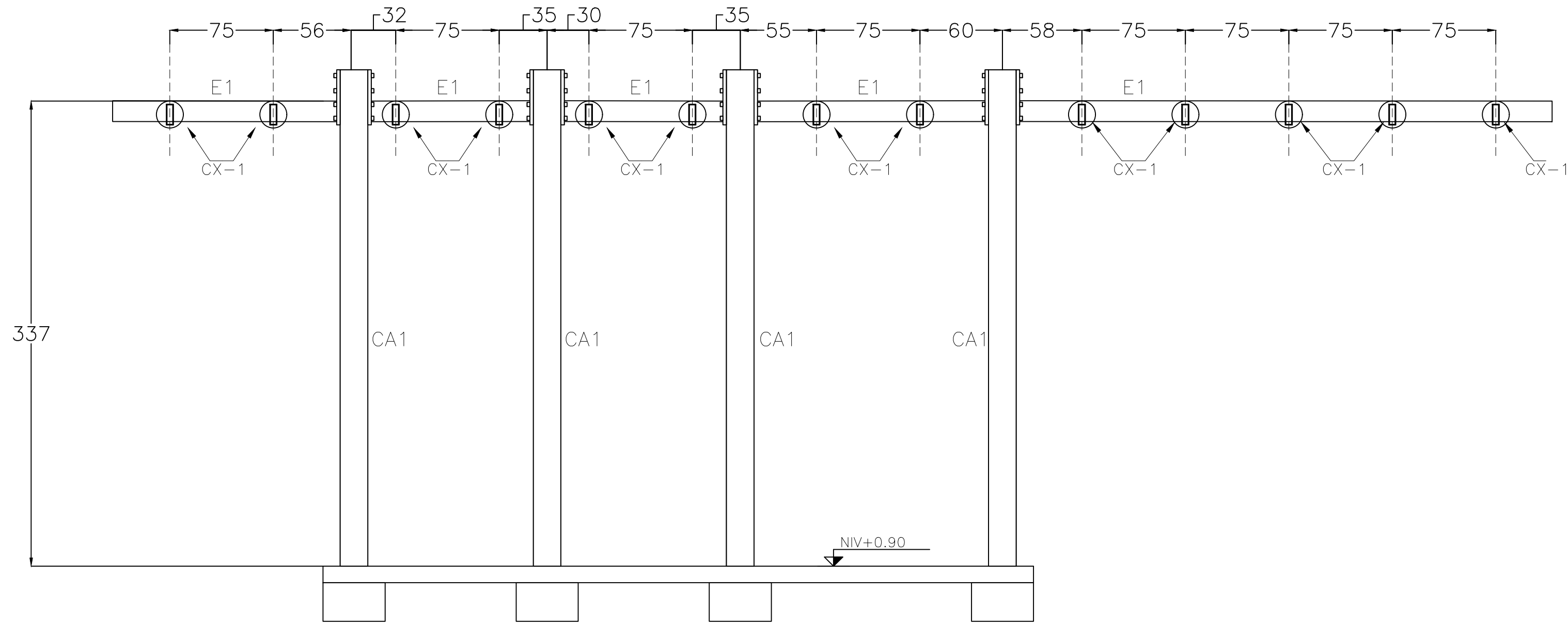
MARCO LONGITUDINAL CUBIERTA 1 Acot: mm
