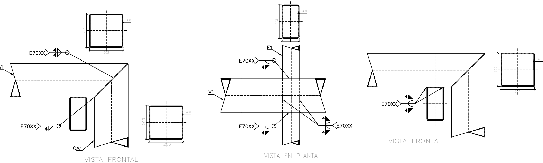
DETALLE CONEXION TIPO CX-3 Acot: mm
