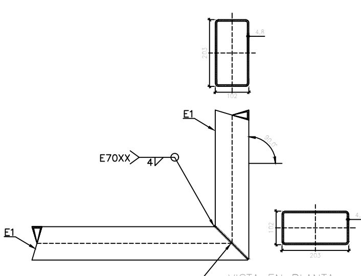
DETALLE CX-2 Acot: mm
