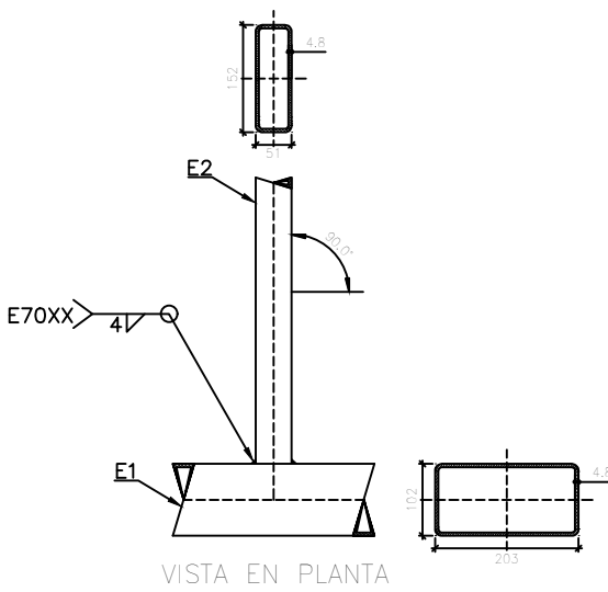
DETALLE CX-1 Acot: mm
