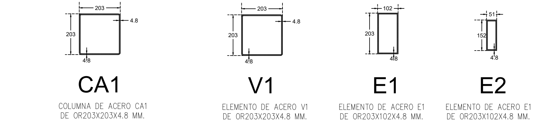
DETALLE COLUMNA CA1 Acot: mm DETALLE ELEMENTOS CUBIERTA Acot: mm
